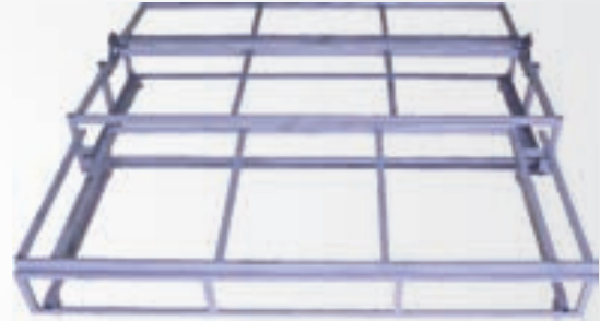
P 4300 000 Öykü İkili Yataklı Kasa Ölçüsü : 800x1380 mm Açık Ölçüsü : 1380x1850 mm
