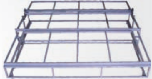
P 4210 000 Öykü Üçlü Yataklı Kasa Ölçüsü : 800x1850 mm Açık Ölçüsü : 1900x1850 mm
